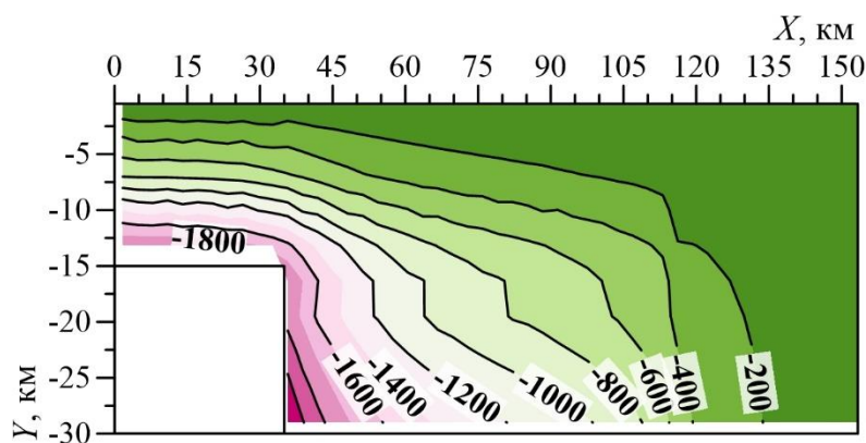
Рис. 5. Распределение термоупругих напряжений
